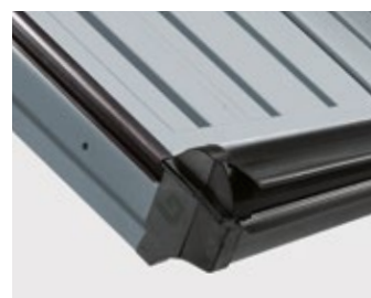
La zoccolatura inferiore in abs, di colore nero, ha una altezza di 50 mm, tappi laterali di chiusura e un profilo di alluminio all'interno. Il risultato estetico pregevole garantisce anche una perfetta chiusura tra anta mobile e pavimento. Optional.
